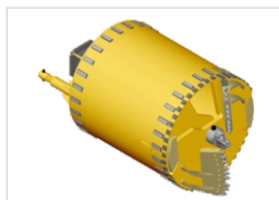
RB-H2 Double Edge Bucket
